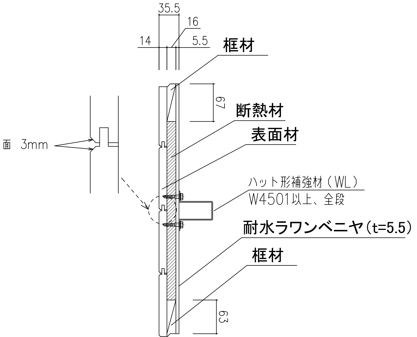
<木製断熱オーバーガレージドア 断面詳細図>
